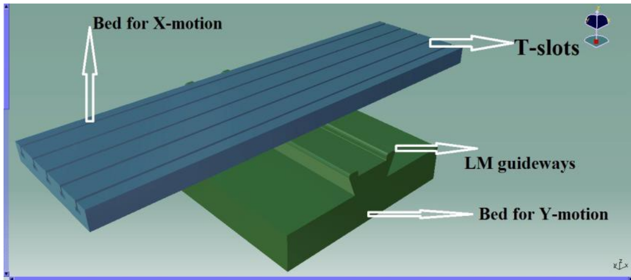
Fig. 18 X-Y table
